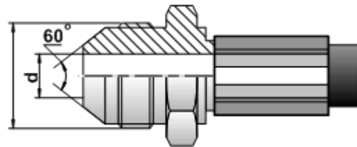
JIS-(Ш) ниппель с наружной резьбой
