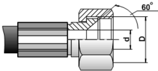
JIS-(Г) фитинг с накидной гайкой
