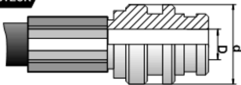
JIS-(Г) фитинг с накидной гайкой
