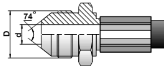
DKI-(Ш) ниппель с наружной резьбой
