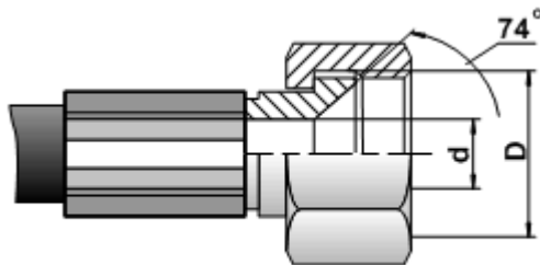
DKI-(Г) фитинг с накидной гайкой
